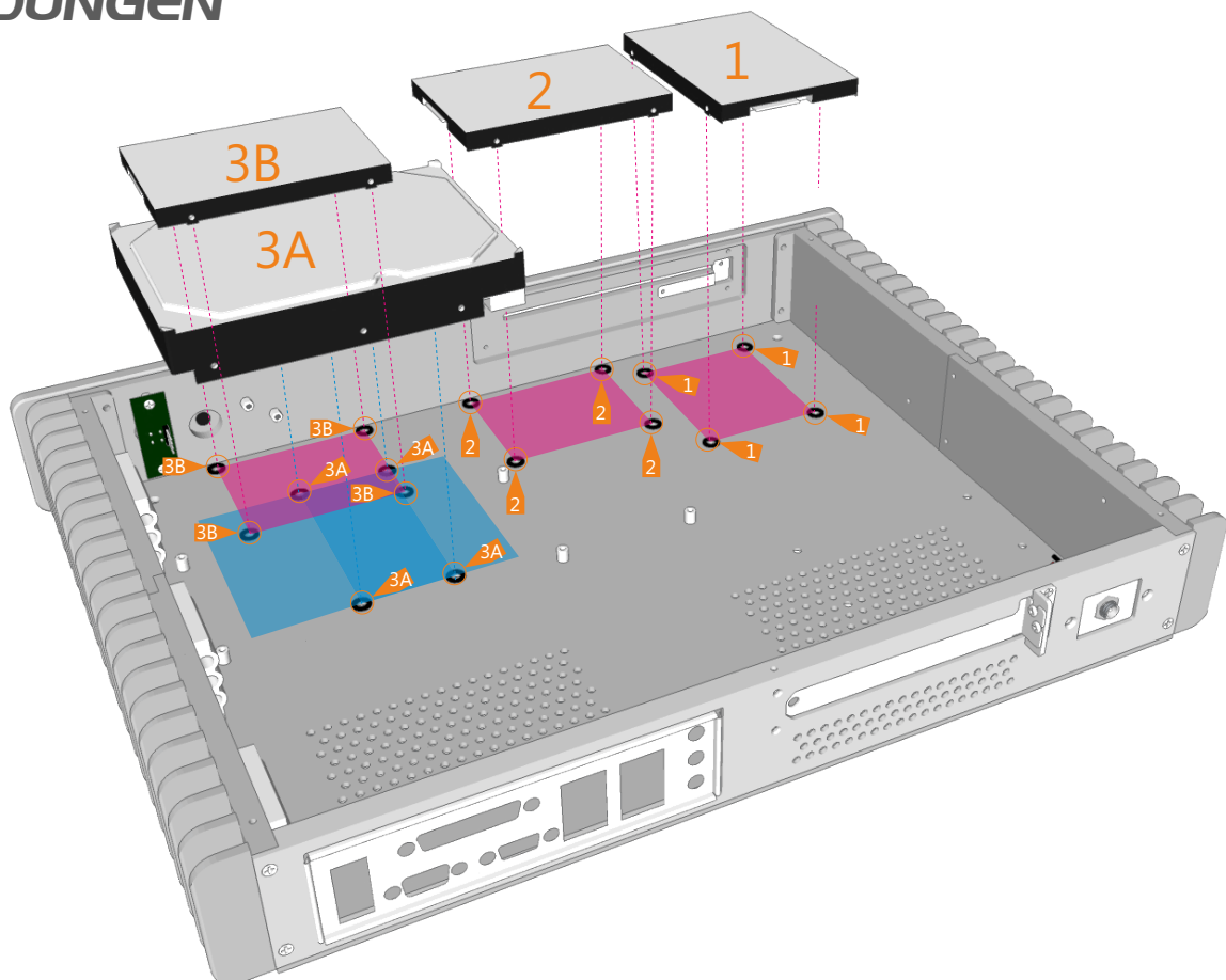
AUSZUG AUS DEM HANDBUCH, ZEIGT DIE INSTALLATION DER LAUFWERKE.
